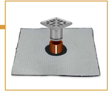
Cód: 4215 (40H), Tubo Diam 40; Porta rejilla 4220
