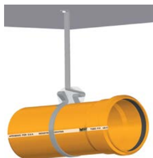
Sujeción simple de tubo Ø 110, fijando la cinta GrampaFlex a la losa, pasando por la hebilla.
